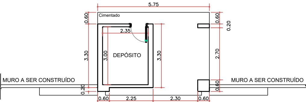
PLANTA ESC. 1:100
