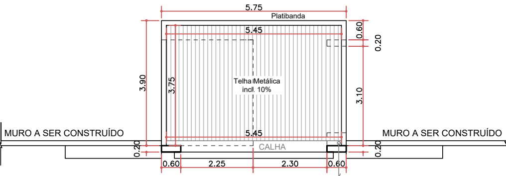
COBERTURA ESC. 1:100
